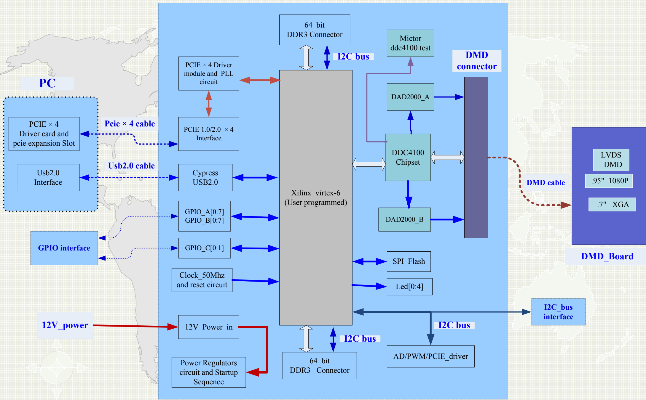
DLP_V6_Pcie_V1.3 Controller Board
